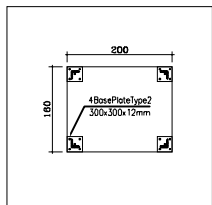
نقشه صفحه گذاری کف جاله آسانور Sc. 1:50
