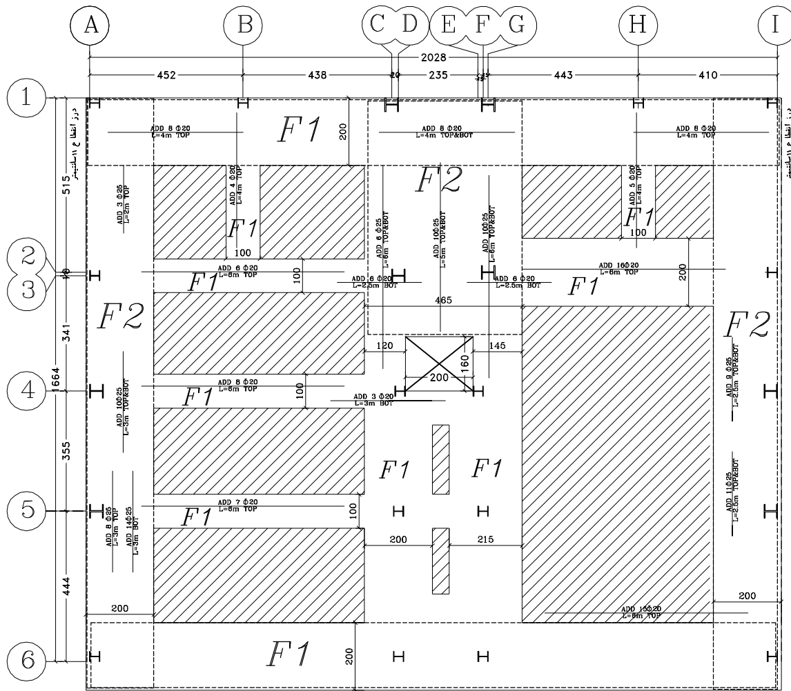
پلان فونداسیون و میلگردهای تقویتی
