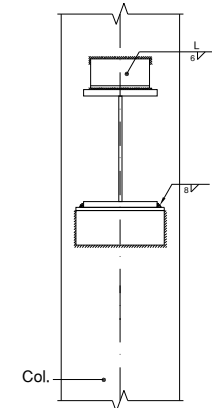
برش 1-1
