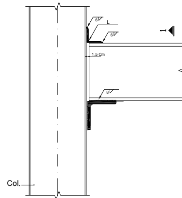
جزئیات اتصال مفصلی تیر به ستون
