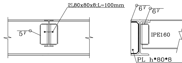
اتصال IPE160 به تیر اصلی
